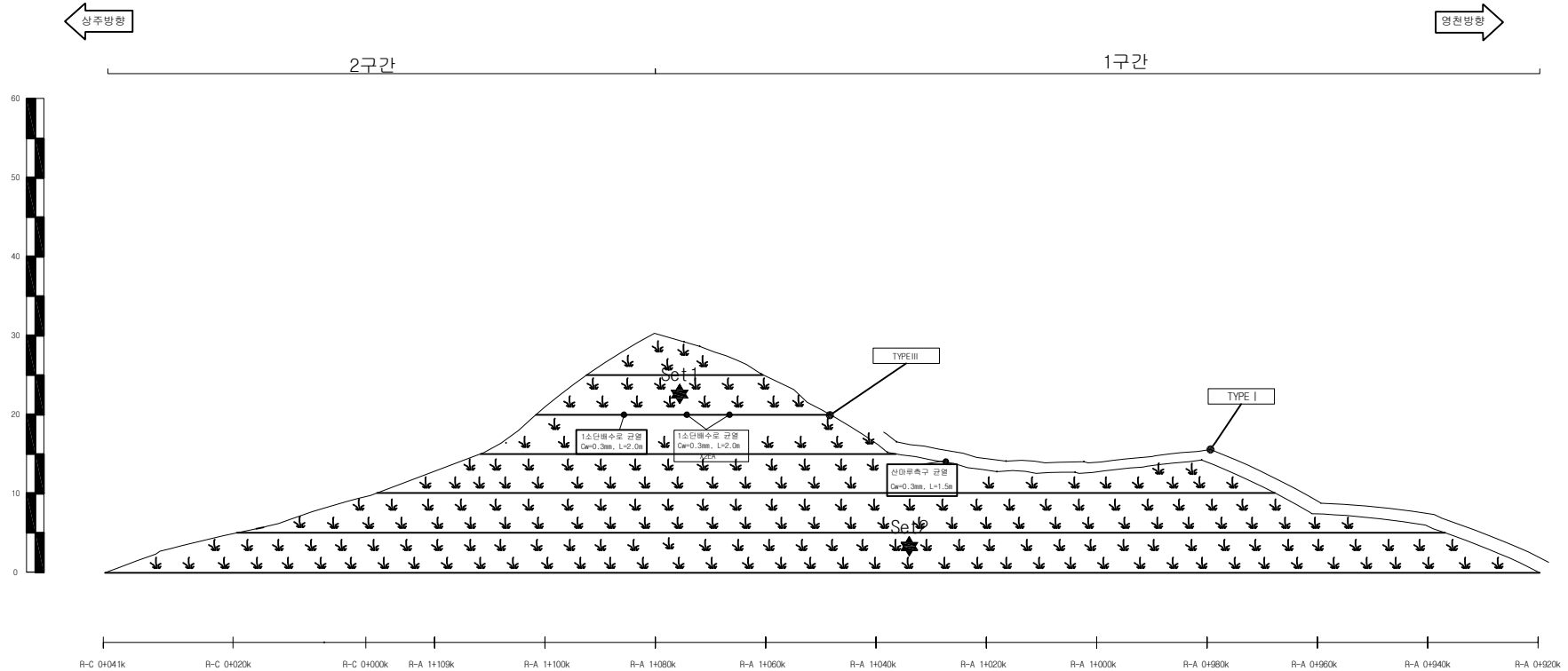
상주절토07 / 관리이정 R-A 0+920~R-C 0+041
