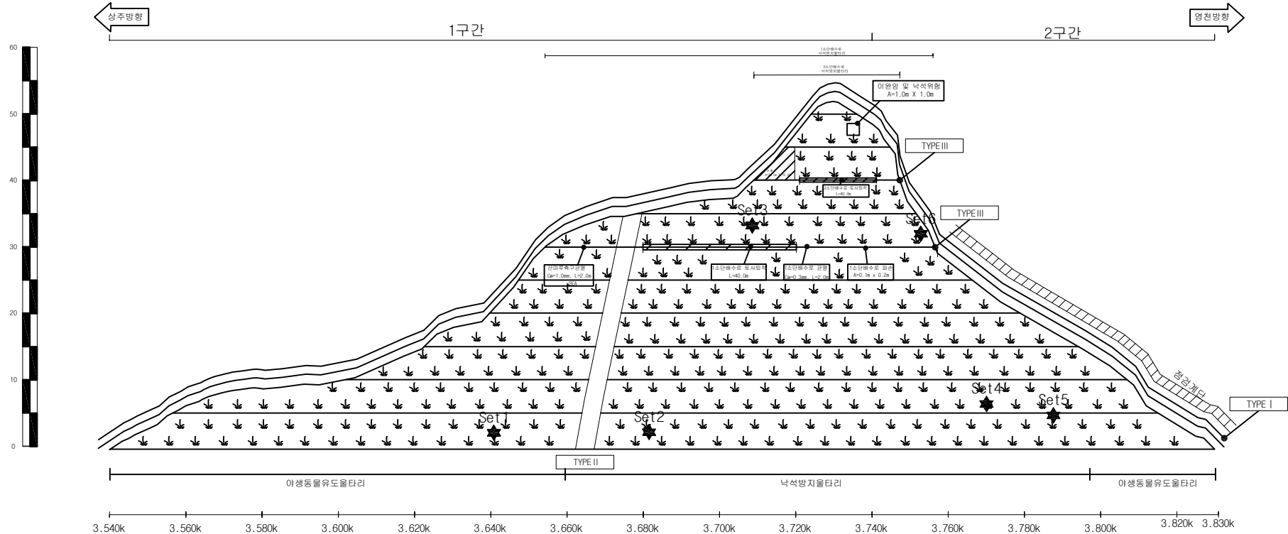
상주절토03 / 관리이정 3.540k~3.830k
